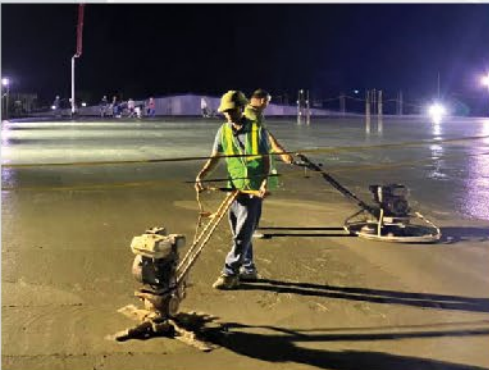
打夯机
